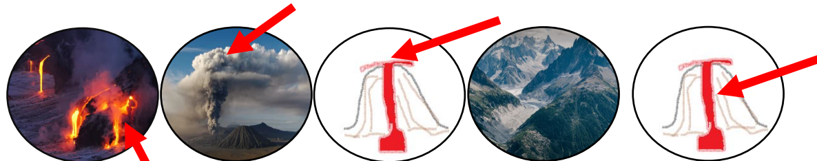
lava ash cloud vent range conduit
